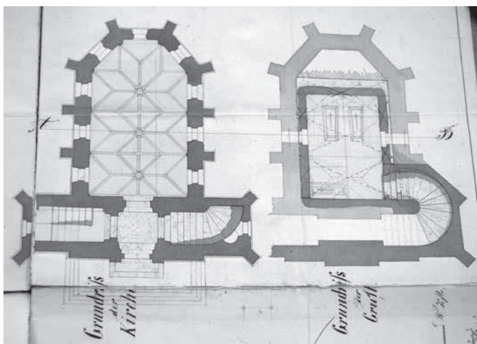
Plán přizemí kaple a krypty (Státní oblastní archiv v Třeboni, Velkostatek Lnáře, inv. č. 1170, sign. V b-7, kart. 17)
